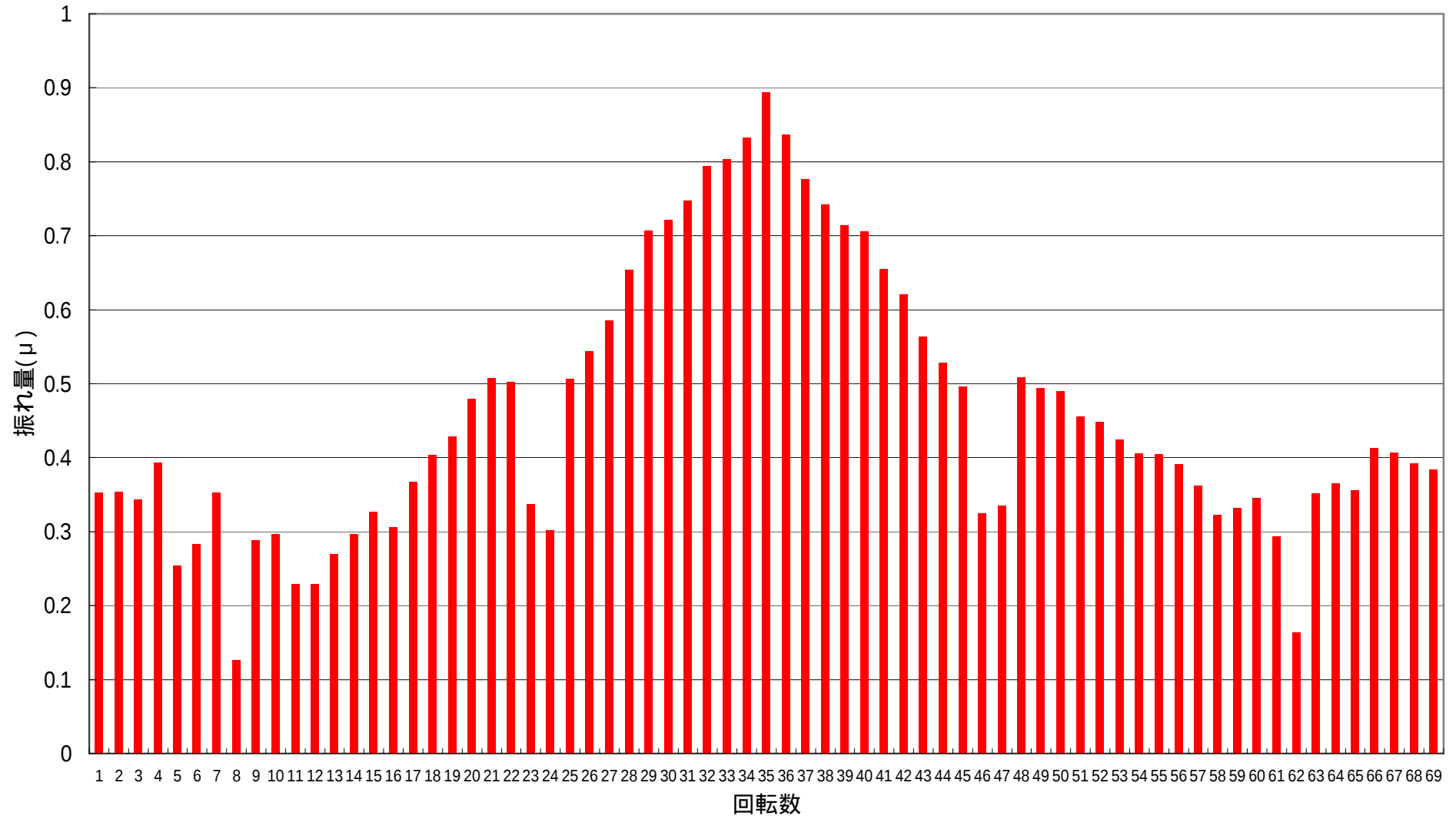
スピンドル回転数別振れ量
